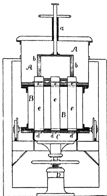
FIG. 19.—Leimdoerfer cooler.
